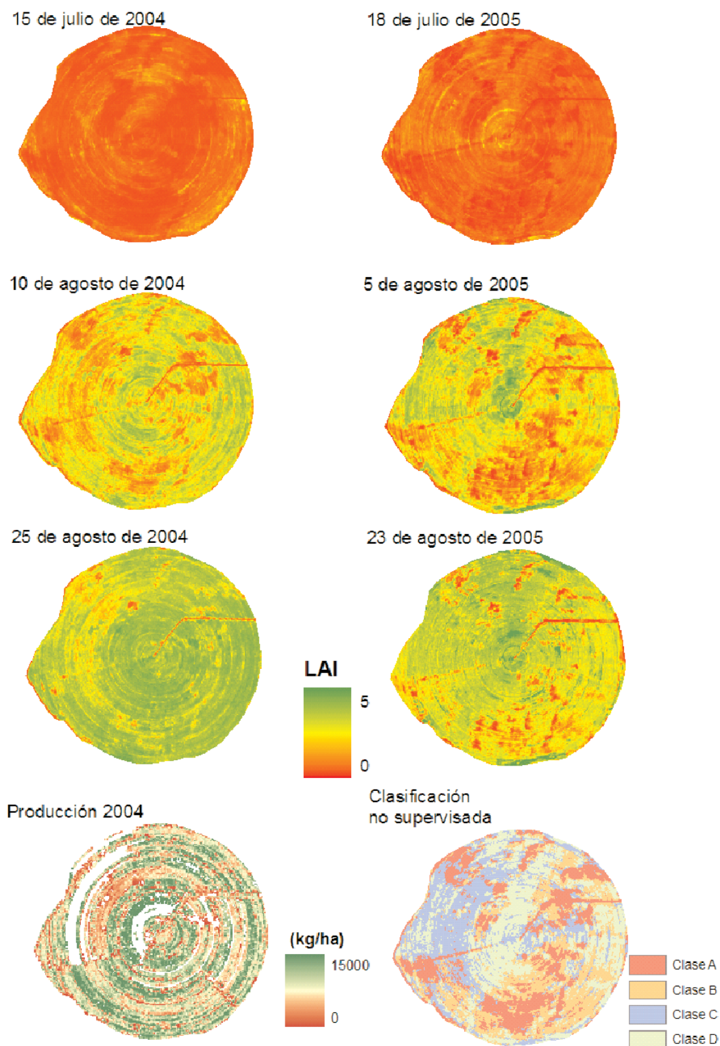
Figura 4. Mapas de LAI generados a partir de las imágenes Quickbird de 2004 y 2005, producción para el año 2004 y clasificación no supervisada a partir de los mapas de LAI del 10 de agosto de 2004 y 5 de agosto de 2005.
