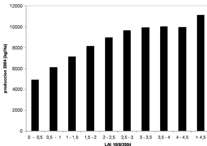
Figura 3. Producción media en 2004 para 10 intervalos del LAI estimado a partir de la imagen del 10 de agosto de 2004.
