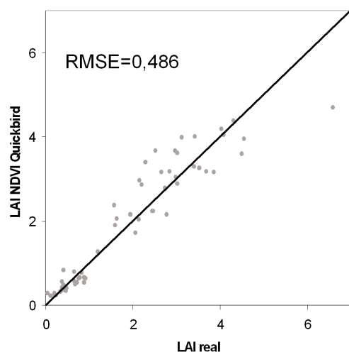
Figura 2. RMSE y diagrama de dispersión para los mapas de LAI obtenidos a partir del NDVI.
