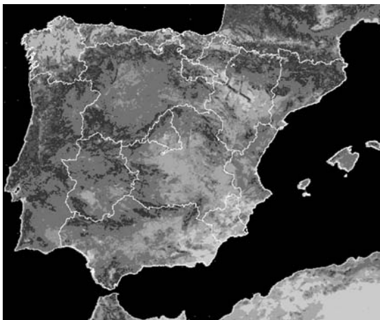
Figura 1. NDVI medio del período 1987-2001.
