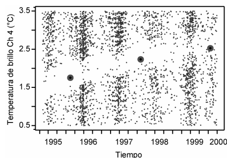
Figura 1: Series temporales de la temperatura de brillo del canal 4 del NOAA-14 AVHRR de la base de datos Pathfinder. Los círculos grandes indican temperaturas de brillo correspondientes al nivel digital 511 (ver texto para explicación).
