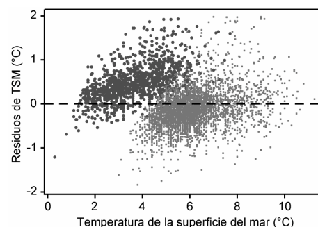
Figura 2: Residuos en función de la TSM in situ para los “matchups” del NOAA-14, periodo 1995–1999. Los círculos negros indican “matchups” con T_4 < 1,5^{\circ}\text{C} . Las cruces grises se corresponden a “matchups” con 3,0^{\circ}\text{C} < T_4 < 5,0^{\circ}\text{C} .
