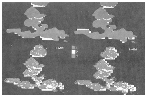
Fig. 4.- Verificación espacial de resultados. la categoría 1 representa los píxeles identificados como incendio en la imagen TM y en el perímetro, pero que no coinciden con la estimación de la imagen NOAA. la categoría 2, en cambio, representa los píxeles que se consideraron como incendios en la imagen, NOAA, pero que no lo fueron en la imagen TM y el perímetro. Por último, la categoría 3, representa los píxeles coincidente entre ambas estimaciones.
