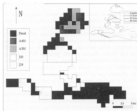
Fig. 3.- Evaluación espacial del incendio. En la esquina superior derecha, perímetro final y evolución del frente de llamas según datos de ICONA
