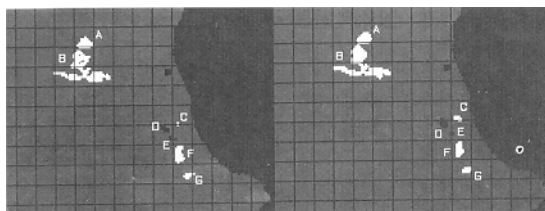
Fig. 2.- Cartografía de áreas quemadas sobre los MVC (izquierda), y sobre los MDVI diarios (derecha).
