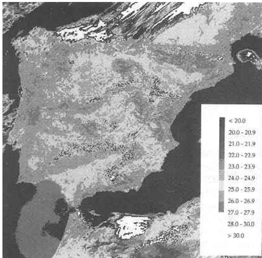
Fig. 3.- Irradiancia solar neta (MJ m -2 d -1 ) 12 junio 1991
