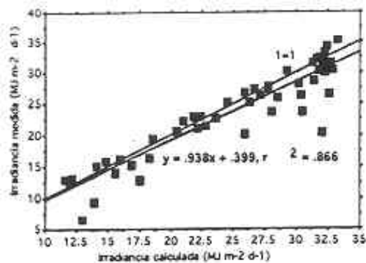
Fig. 1.- Irradiancia calculada Vs. Irradiancia medida (MJ m 2 d -1 ) HOBART, TASMANIA 42.8°S 147.2°E
