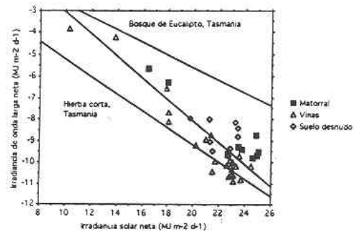
Fig. 4.- La traza de L^* Vs. K^* en varios lugares (MJ m -2 d -1 )
