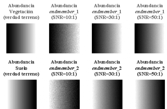
Figura 2. Mapas de abundancia verdad terreno y valores de abundancia estimados por AMEE en presencia de diferentes valores de SNR.
