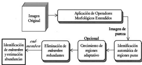
Figura 1. Diagrama de bloques que resume el funcionamiento del método propuesto.
