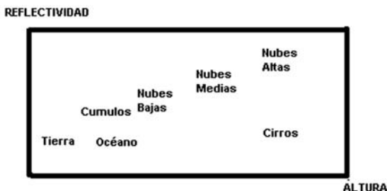
Figura 2. Reflectividad vs. altura
