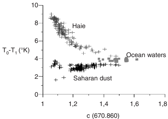
Figura 2. Diagrama de dispersión entre \Delta T_{4,5} (ordenadas) y el parámetro \epsilon_{1,2} (abscisas) para mostrar la separabilidad entre los fenómenos presentes en las escenas.
