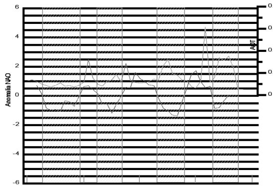
Figura 4. Serie temporal de espesor óptico superpuesta a la anomalía estandarizada del índice NAO para el período 1997-2000. Sombreado en azul los períodos negativos de la NAO.
