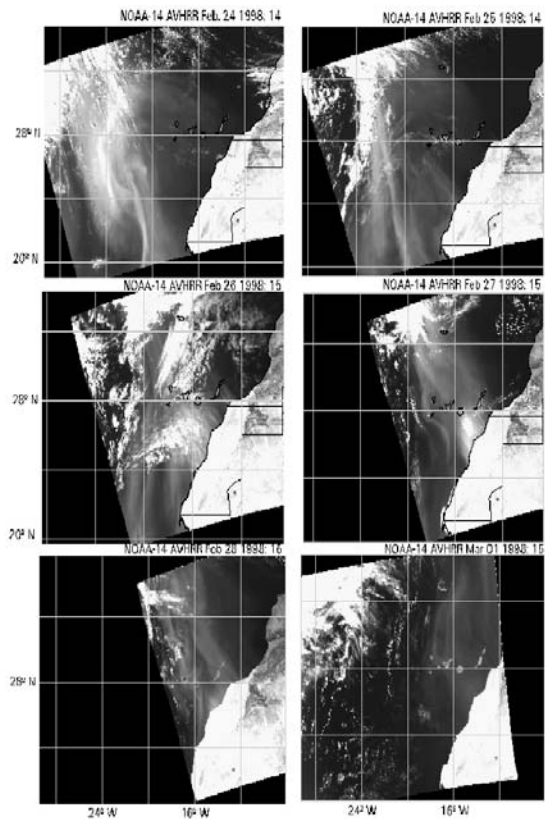
Figura 1. Secuencia de imágenes AVHRR, del 24-02 al 01-03 de 1998, mostrando la evolución de una lengua de polvo sahariano en la zona de Canarias. RGB = Reflectancia canal 1, idem canal 2 y temperatura del brillo canal 4.
