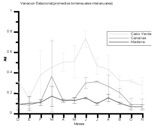
Figura 5. Variación estacional para el período 1998-2000.
