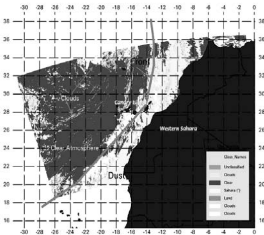
* Figura 3. Clasificación de la imagen AVHRR del 15-02-98 en base a las transformaciones de la figura 2. Mostrando la separabilidad entre océano, nubes, aerosoles y tierra.
