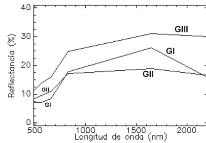
Figura 4.- Perfiles espectrales correspondientes a los grupos espectrales de la figura 3, extraídos de la imagen TM calibrada.
