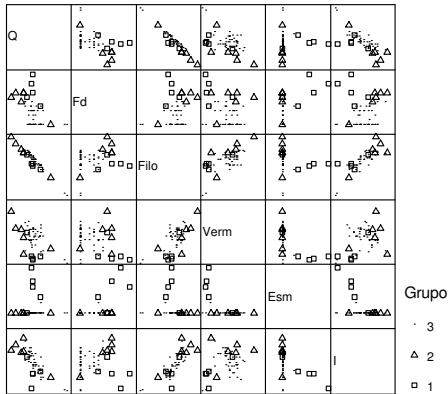
espectrales en Figura 2.- Relaciones entre los distintos minerales presentes en las muestras estudiadas y los grupos espectrales a los que dichas muestras han sido asignadas. (Q: cuarzo, Fd: feldespatos, Filo: filosilicatos, Verm: vermiculita, Esm: esmectitas, I: illita).
