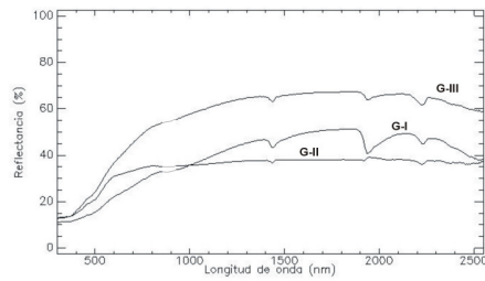
Figura 3.- Curvas espectrales de laboratorio representativas de los tres grupos diferenciados.
