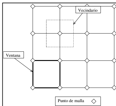
Figura 2. Esquema del método de interpolación adaptativo bilineal.
