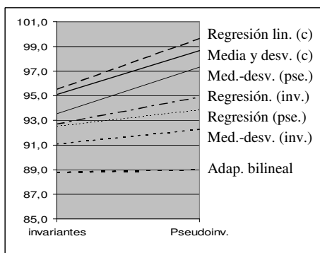
Figura 3. Comparación de los resultados del ensayo 1 para el solape 1-3. Tipos de muestras: invariantes (inv), pseudoinvariantes (pse), imagen completa (c).
