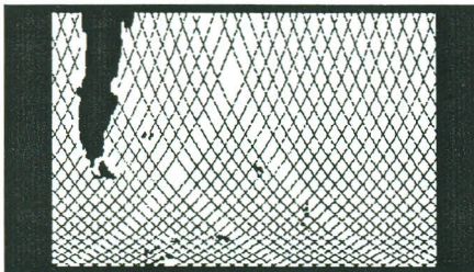
Figura 6.- Las órbitas del satélite TOPEX-POSEIDON tienen una alta estabilidad de repetición espacio-temporal en sus ciclos de 10 días, sobrevolando las mismas áreas geográficas. En la figura se presentan los pasos orbitales 7, 11, 061, 111, 163, 237, 239. Los puntos de corte de las órbitas ascendentes y descendentes se mantienen dentro de un círculo de 1Km a lo largo de la misión con la finalidad de permitir los estudios de variación temporal en esos puntos a lo largo de la misión.
