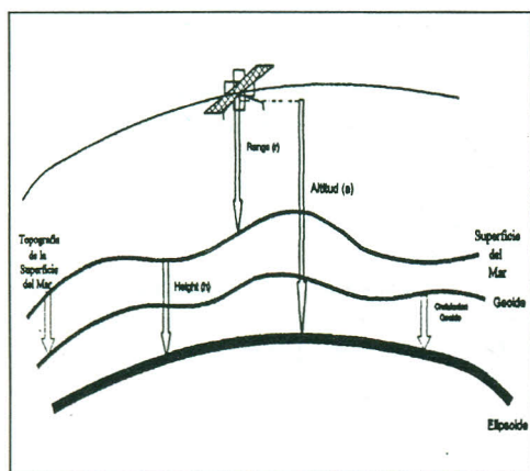
Figura 2.- El altímetro del satélite mide la altura del satélite sobre el océano con precisión centimétrica. La ecuación que relaciona la medida del altímetro " r " (range) con la altitud " a " y la altura " h " sobre elipsoide de referencia del nivel del mar (height) y las correcciones a la medida debidas al entorno es: \text{NIVEL DEL MAR (h)} = \text{ALTITUD(a)} - \text{ALTURA Altímetro(r)} + (\text{CORRECCIONES: Atmosféricas (ionosfera y troposfera), Oleaje, Lluvia, Mareas (oceánicas y terrestre), Movimiento del Polo, Barómetro Invertido}). Si se desea obtener la topografía dinámica del océano hay que restar al nivel del mar(h) obtenido, las ondulaciones del geoid considerando al geoid como superficie de equilibrio del océano. La topografía dinámica del océano es en estas condiciones: \text{TOPOGRAFIA DINAMICA DEL OCEANO} = \text{NIVEL EL MAR} - \text{ONDULACIONES DEL GEOIDE}
