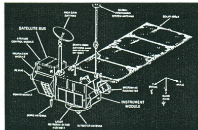
Figura 1.- El satélite TOPEX-POSEIDON se encuentra diseñado para desarrollar la misión altimétrica de mayor precisión hasta la fecha. La órbita del satélite y los formalismos de corrección alcanzando exactitud centimétrica.
