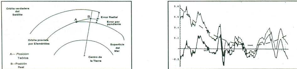
Figura 3.- La figura presenta las salida gráfica del programa ERRORAD referida a la órbita 111 que atraviesa el Mar de Drake ascendiendo para atravesar el arco del "Scotia" entre Malvinas y Georgia del sur. El gráfico izquierdo representa el error radial de la órbita calculada y cuyo error se transmite a la medida altimétrica. El gráfico derecho presenta la corrección efectuada considerando que el geode no presenta deformación espacio-temporal y que la deriva registrada, a lo largo del perfil, en la topografía del océano se debe a errores en la determinación de la órbita que pueden corregirse ajustando un polinomio a los residuos.
