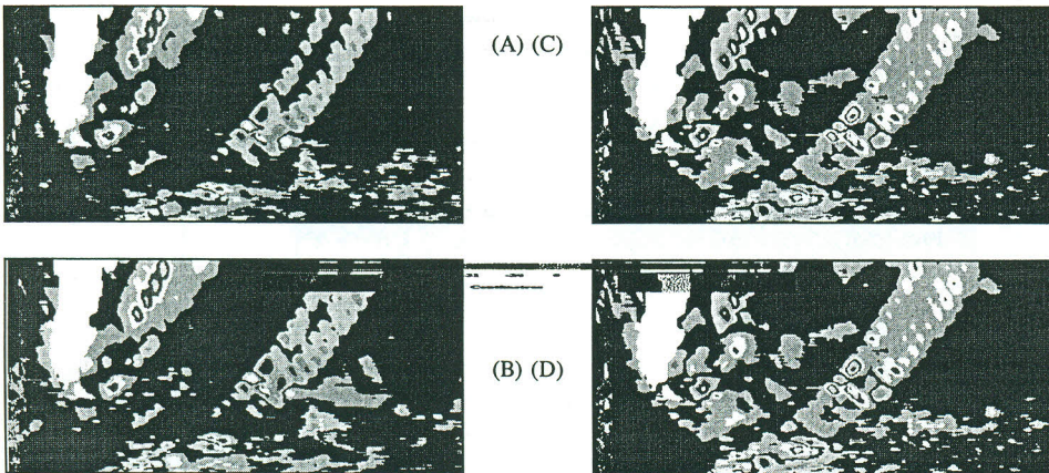
Figura 9.- Variaciones estacionales de la Topografía dinámica del océano. (A)Primavera, (B)Verano, (C)Otoño, (D)Invierno. Puede observarse que las situaciones se repiten en Primavera-Verano y Otoño-Invierno, presentándose en (A), (B) una situación anticiclónica al norte de las Islas Sandwich y una ciclónica al norte de Malvinas. Durante (C), (D) la situación aparece invertida. (C.20)
