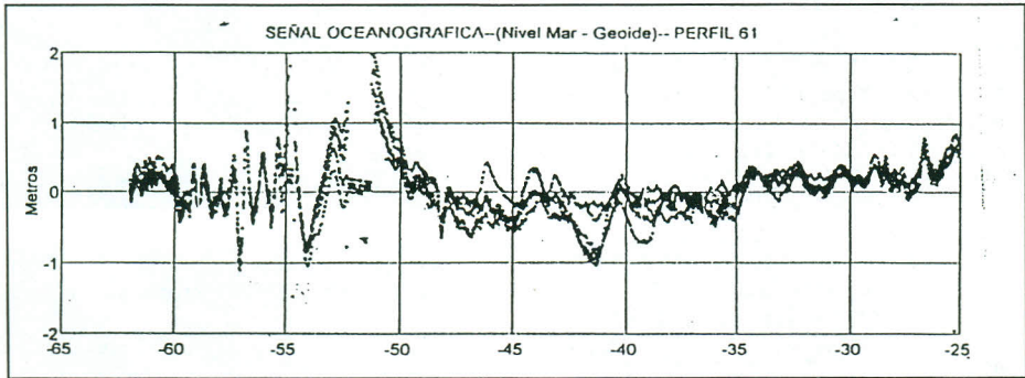
Figura 10.- El perfil 061 cruza el Drake sobrevolando las islas Malvinas hacia Brasil. En la figura se presenta la variación del Nivel del Mar entre Septiembre y Noviembre de 1993 entre 46° y 42ª Sur variaciones en el orden del metro relacionadas con los " eddies" que cruzan la zona entre Malvinas y la Península Valdes.
