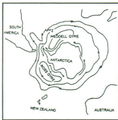
Figura 4.- La figura representa la corriente circumpolar que fluye alrededor del continente Antártico. De norte a sur la zona esta cruzada por los frentes: Subtropical (STF), Antártico (SAF), Polar (PF) y el Agua Costera de Contorno (CWB). Nowling (1986), habiéndose sugerido recientemente un segundo frente entre PF y CWB. Orsi (1993).
