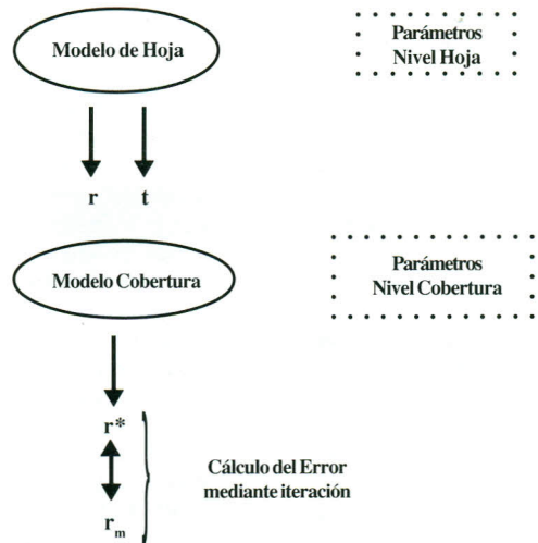
Figura 3. Unión de modelos de transferencia radiativa a nivel de hoja y de cobertura para su inversión ( r^*=p estimada; r_m=p medida).
