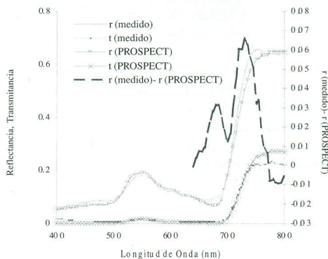
Figura 1. \rho y \tau de acículas medidas mediante el método de Harron & Miller y simuladas mediante el modelo PROSPECT ( chl_{a+b}=68.5 mg/cm 2 , N=3.5).
