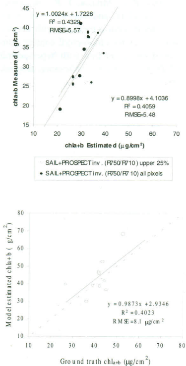
Figura 4. Estimación de contenido clorofílico en zonas forestales de Acer saccharum (arriba) y Pinus strobus (abajo) mediante inversión de modelos PROSPECT, SAILH y SPRINT con datos hiperspectrales del sensor aerotransportado CASI.
