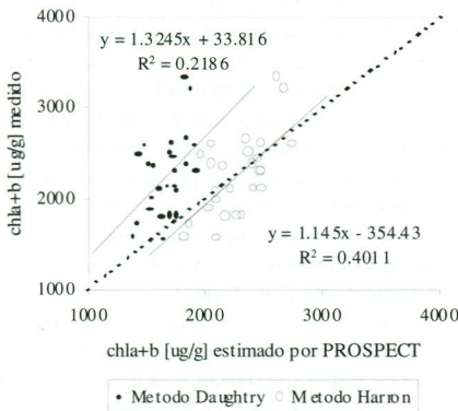
Figura 2. Estimación del contenido clorofílico en acúlas de Pinus strobus mediante inversión del modelo PROSPECT con datos de \rho y \tau medidos mediante el método de Daughtry, y Harron & Miller.
