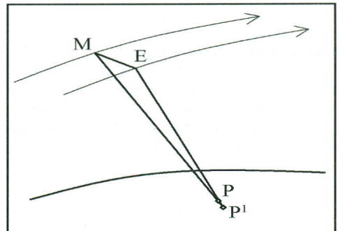
Figura 1. Geometría de la interferometría SAR.
