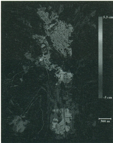
Figura 2. Mapa de subsidencia sobre la zona de Sallent (Barcelona). \Delta T = 981 días.
