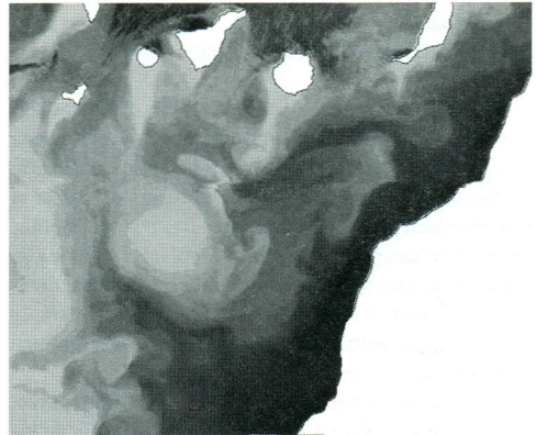
Figura 1. Imagen AVHRR de temperatura superficial ecualizada (10-8-1993).
