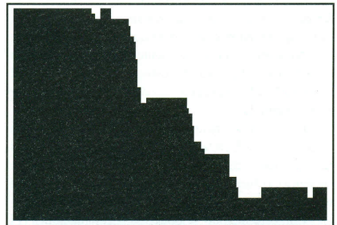
Figura 8. Perfil de la función de imagen (temperatura de brillo).
