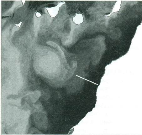
Figura 5. Sección transversal del afloramiento.
