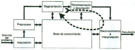
Figura 9. Realimentación de la fase de segmentación.
