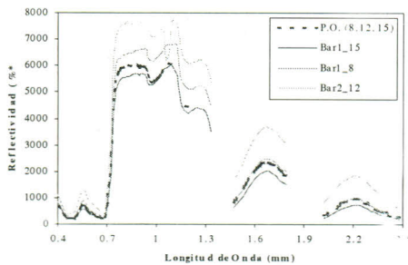
Figura 4. Signatura espectral del pivot de alfalfa bajo diferentes configuraciones de observación.
