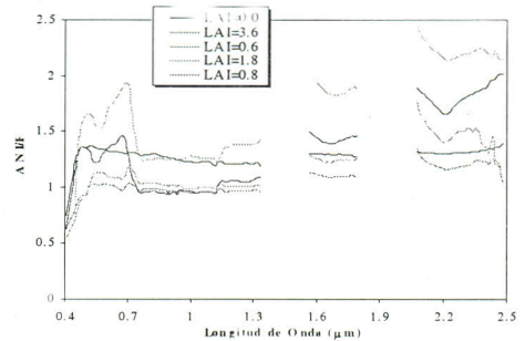
Figura 5. Factor de Anisotropía obtenido entre la imagen de la mañana y del mediodía en el P.O.
